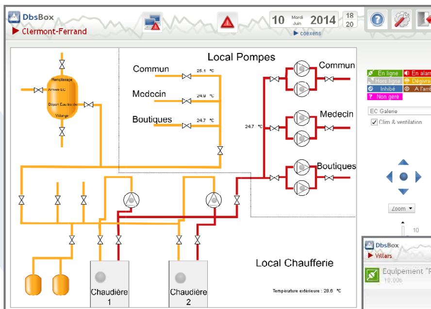
Synoptique dynamique avec indicateurs d'états et principales variables
